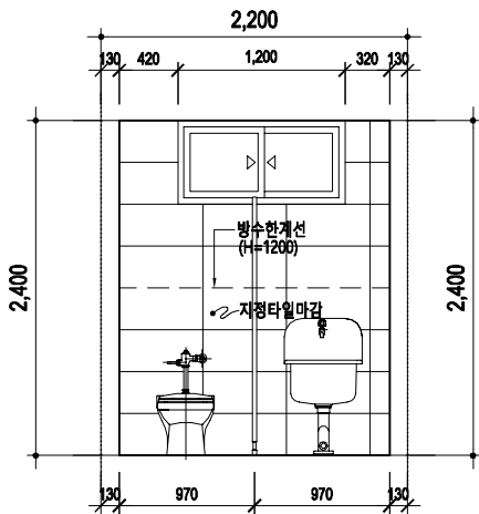
화장실(남) "B"전개도
