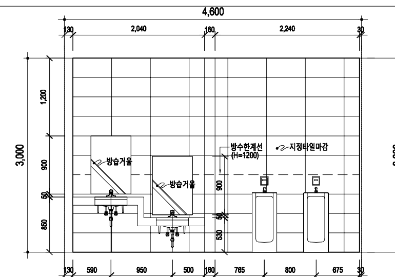
화장실(남) "D"전개도
