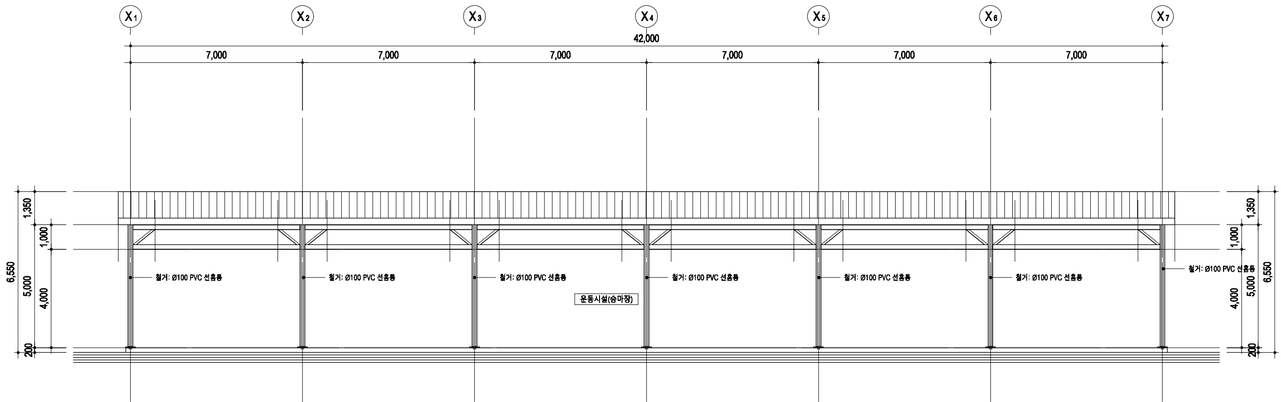
정면도(철거) 축척 A1:1/75, A3:1/150
