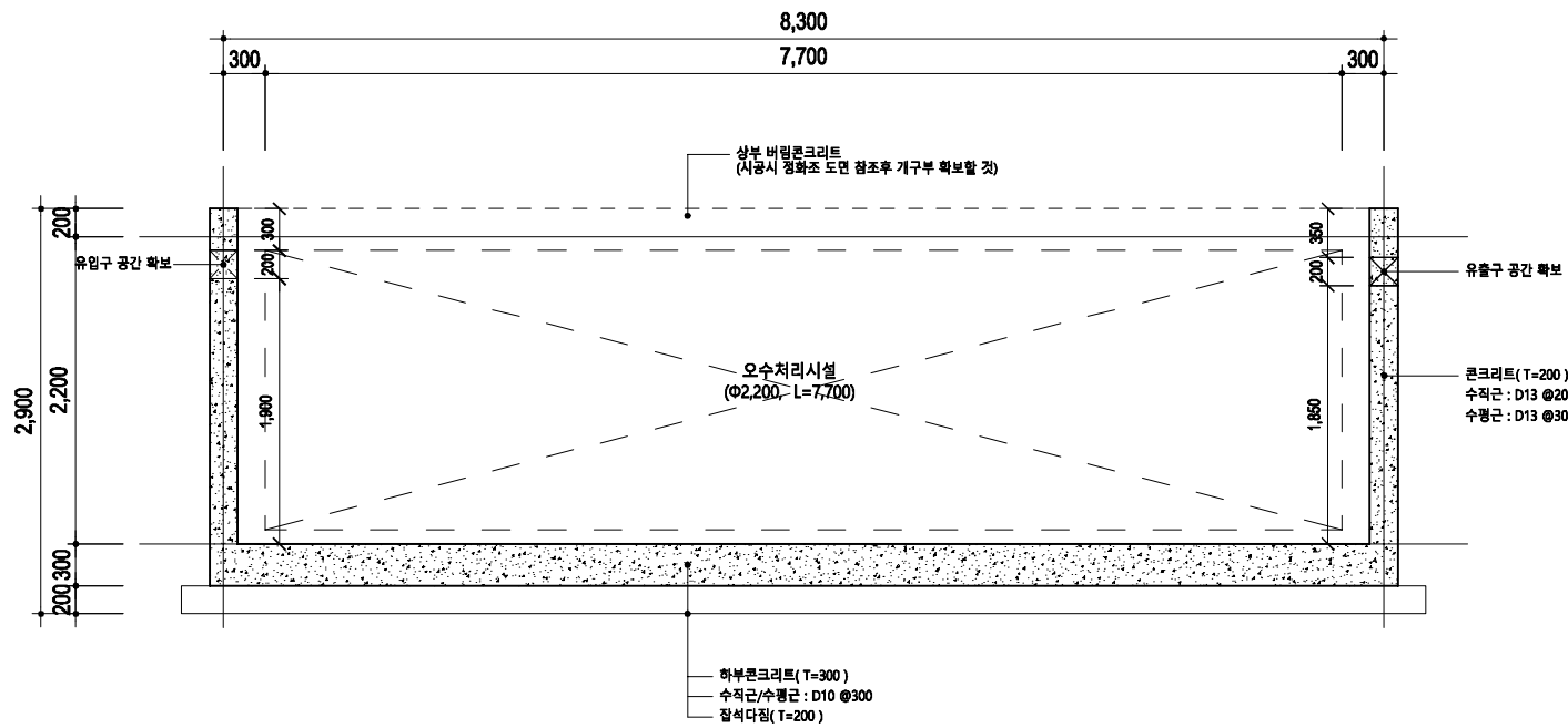
A 단면도
