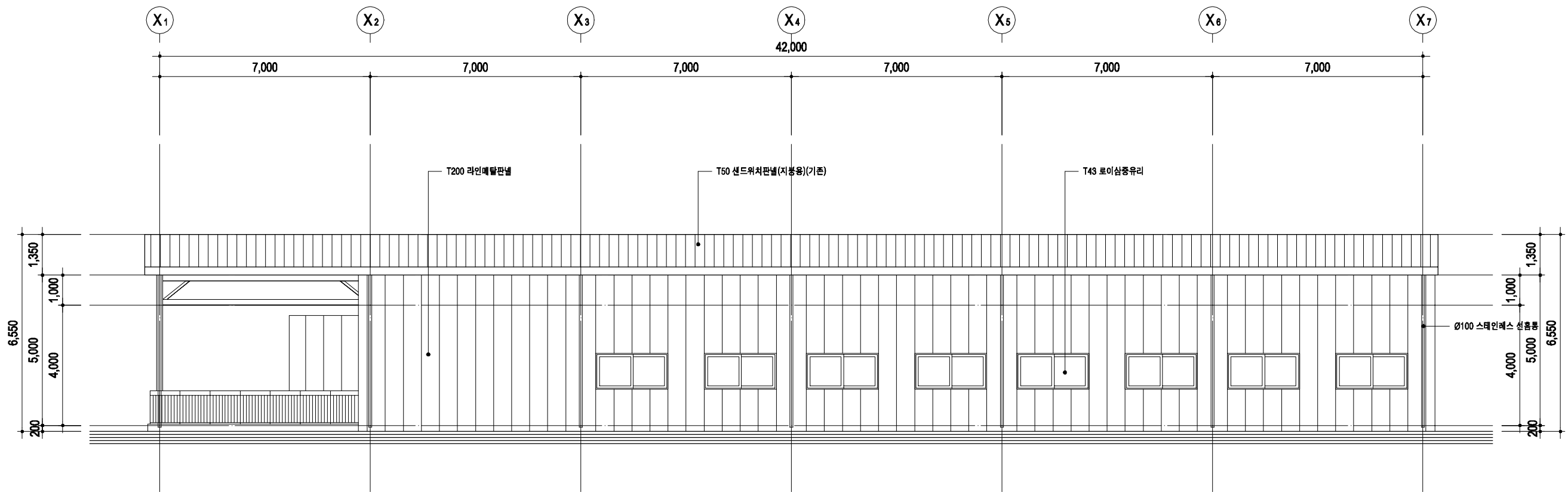
정면도 축척 A1:1/75, A3:1/150
