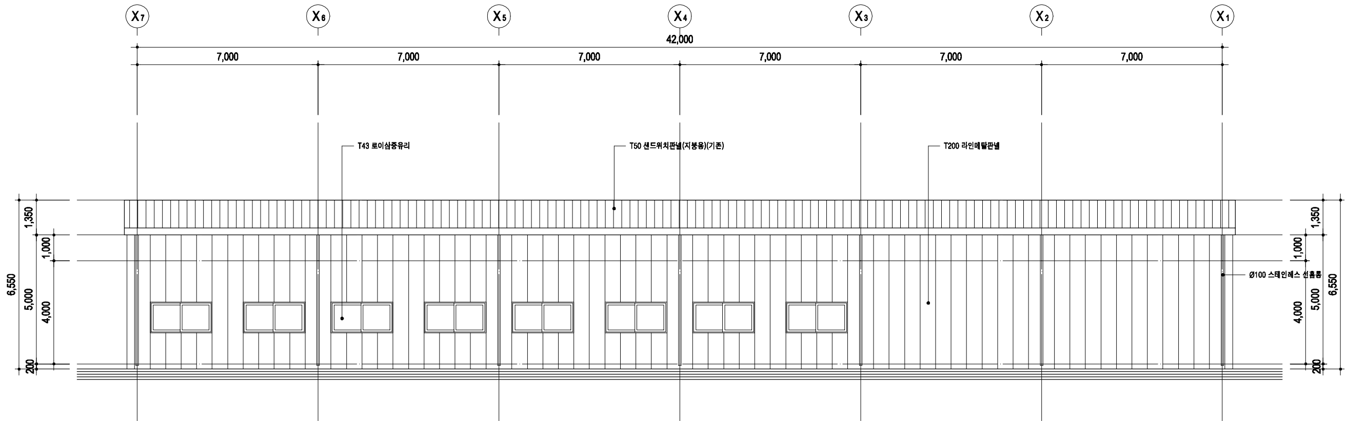
배면도 축척 A1:1/75, A3:1/150
