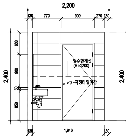
화장실(여) "G"전개도
