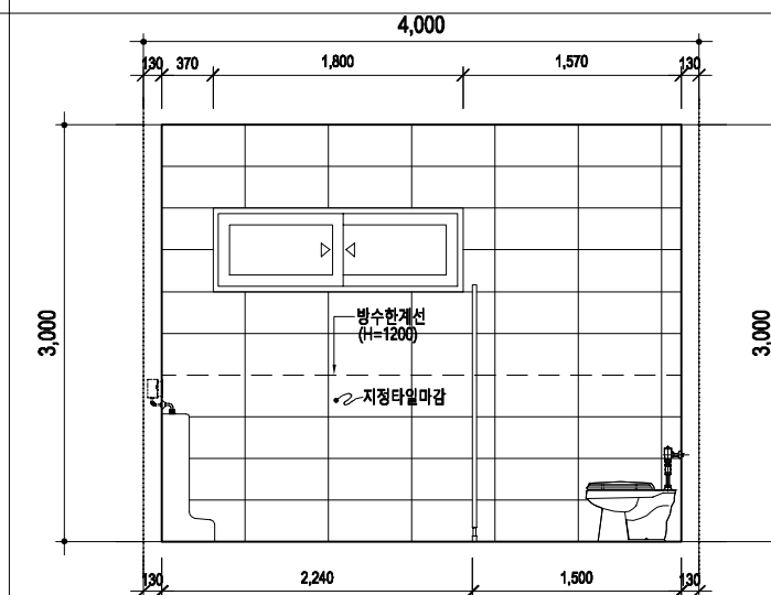
화장실(남) "D"전개도
