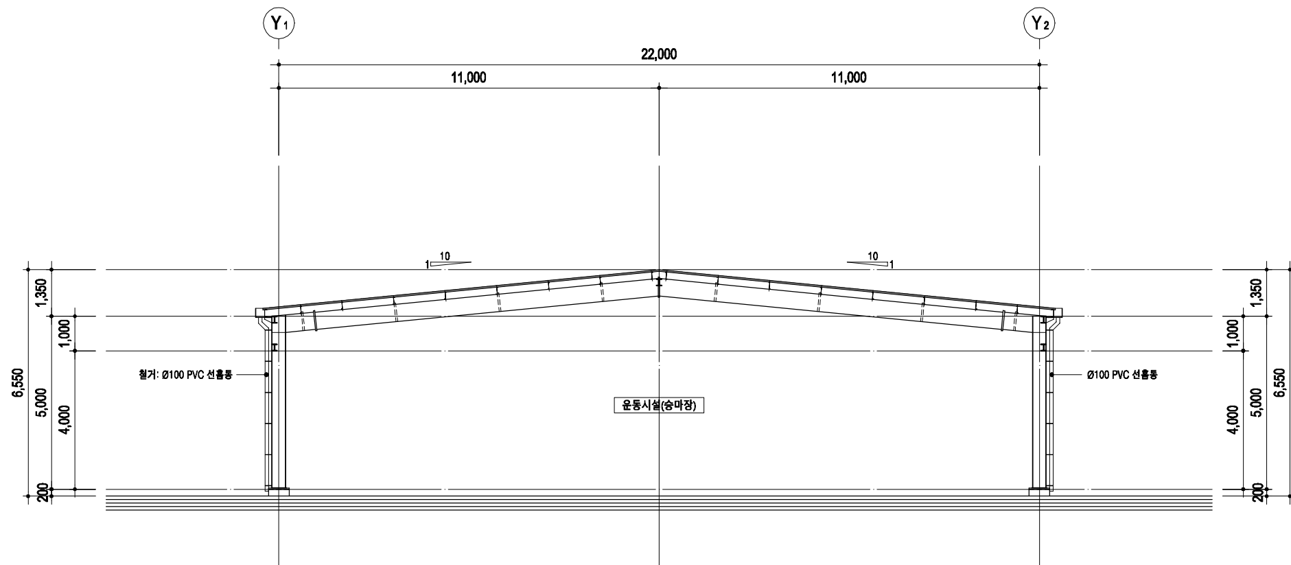
우측면도(철거) 축척 A1:1/75, A3:1/150
