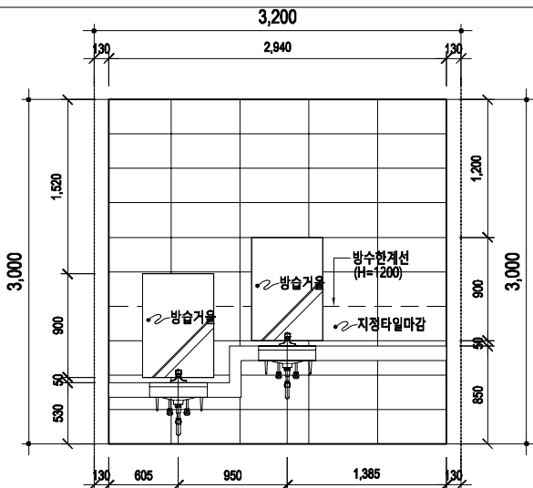
화장실(여) "C"전개도
