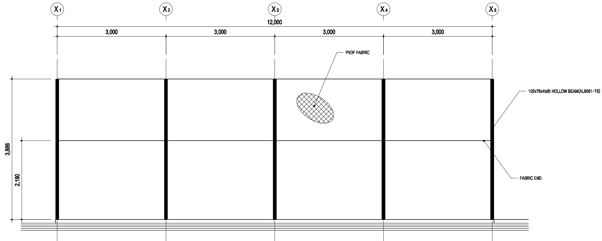
부1- 'A' 정면도(철거) 축척 A1:1/30, A3:1/60
