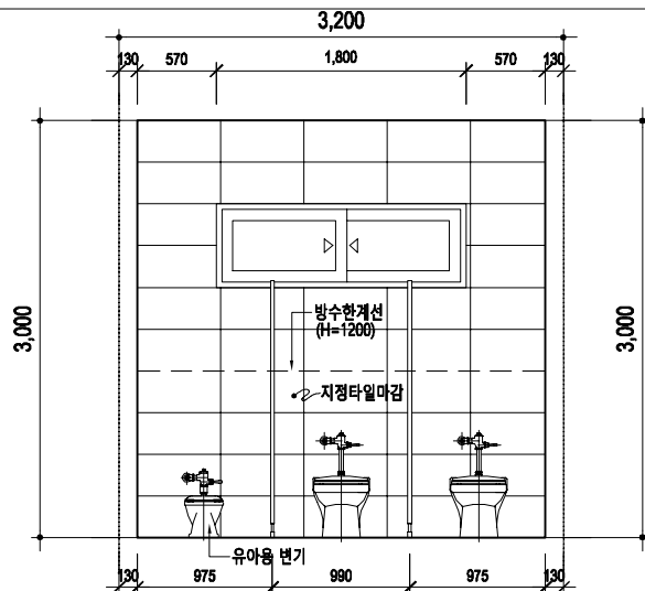
화장실(여) "D"전개도
