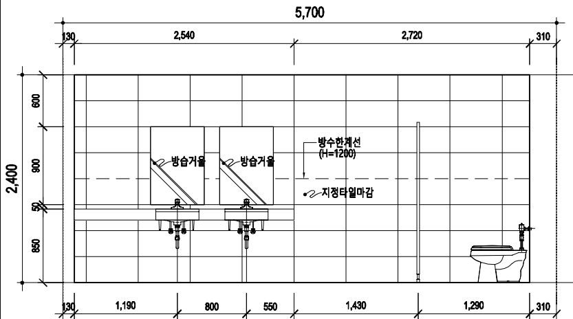
화장실(남) "A"전개도
