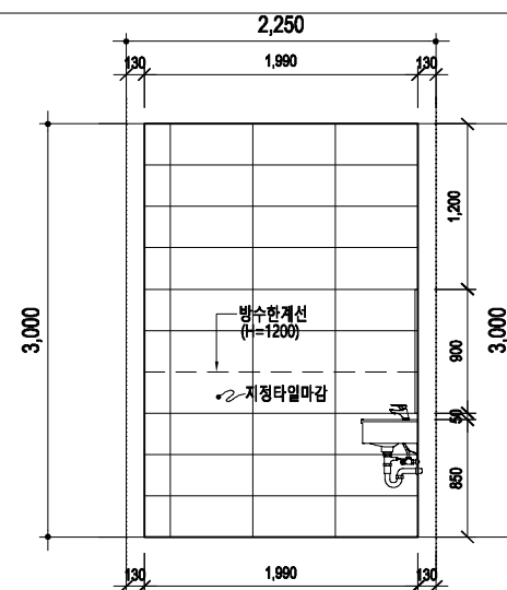
화장실(남) "C"전개도
