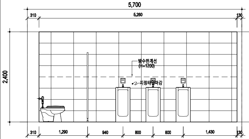
화장실(남) "C"전개도
