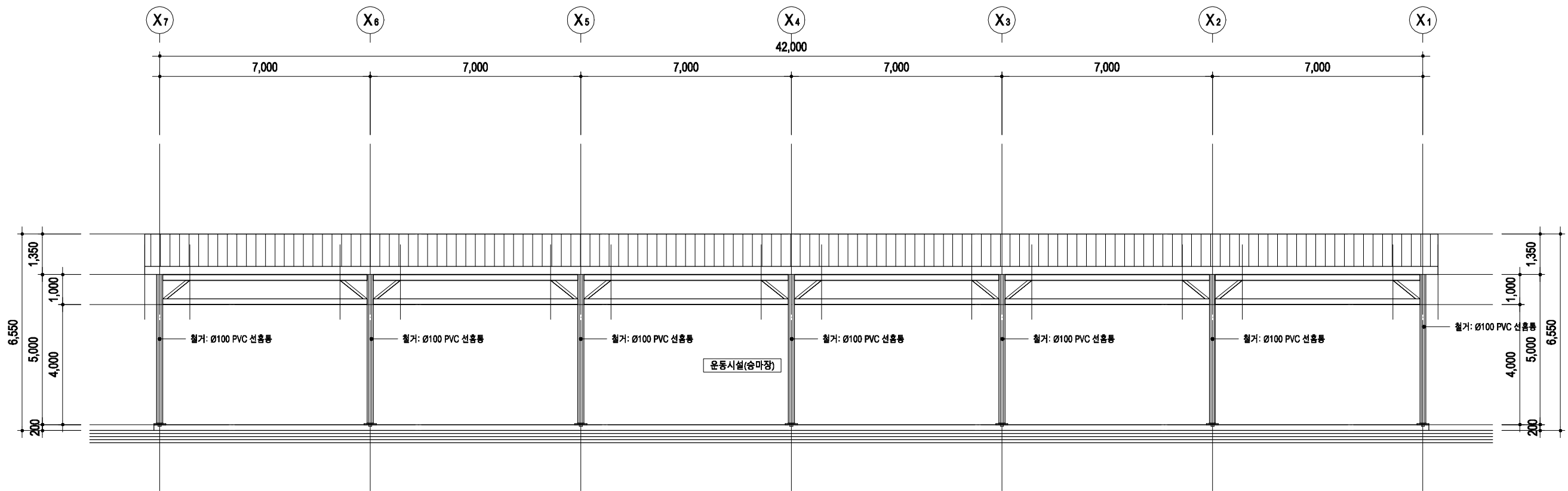
배면도(철거) 축척 A1:1/75, A3:1/150
