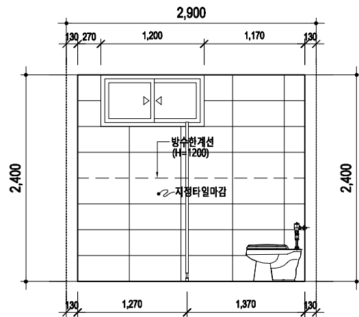
화장실(여) "F"전개도
