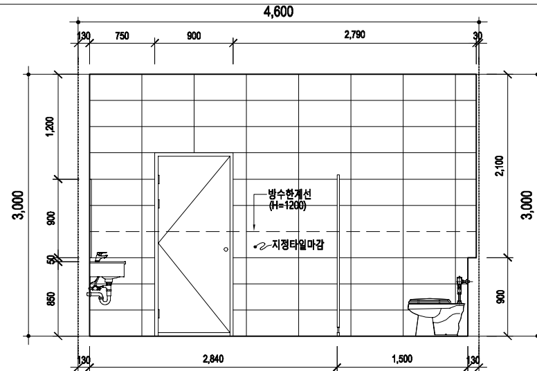
화장실(여) "D"전개도
