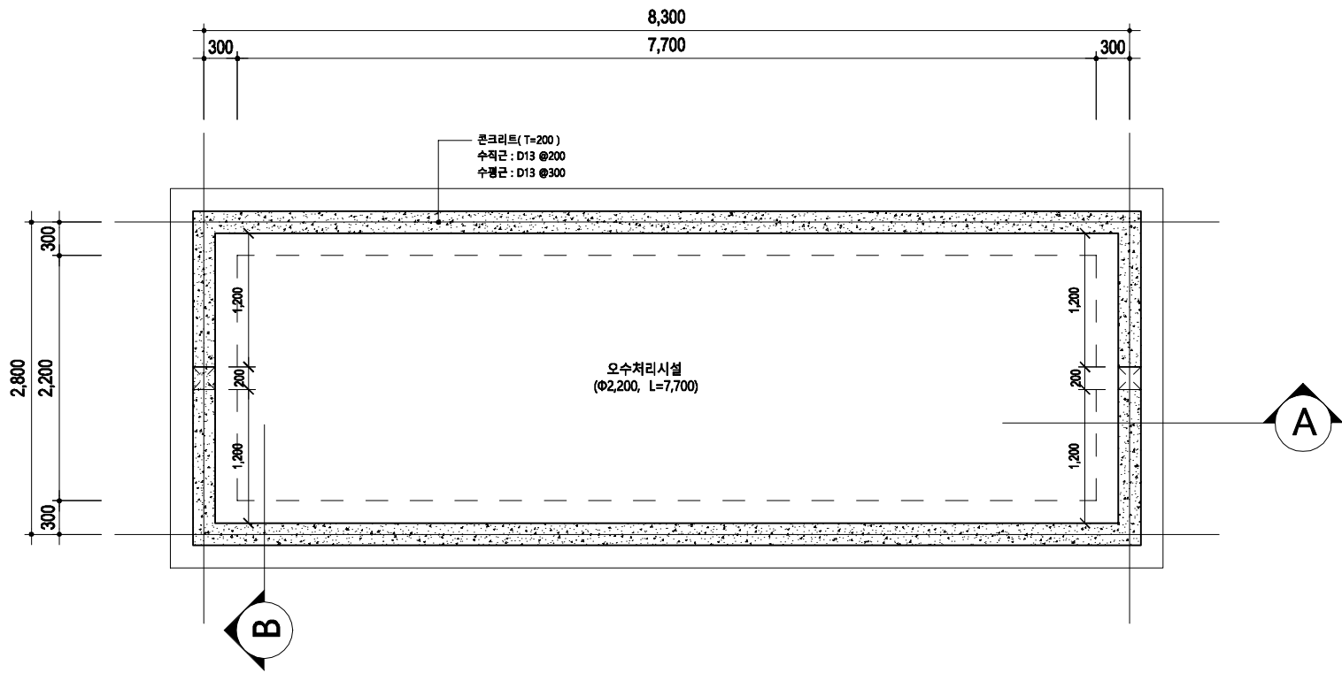
평면도
