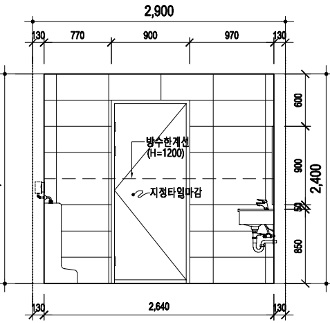
화장실(남) "D"전개도
